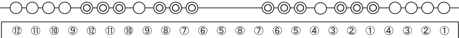
第1サスペンションライト フライダクト T型20Aコンセント 12回路 24個
