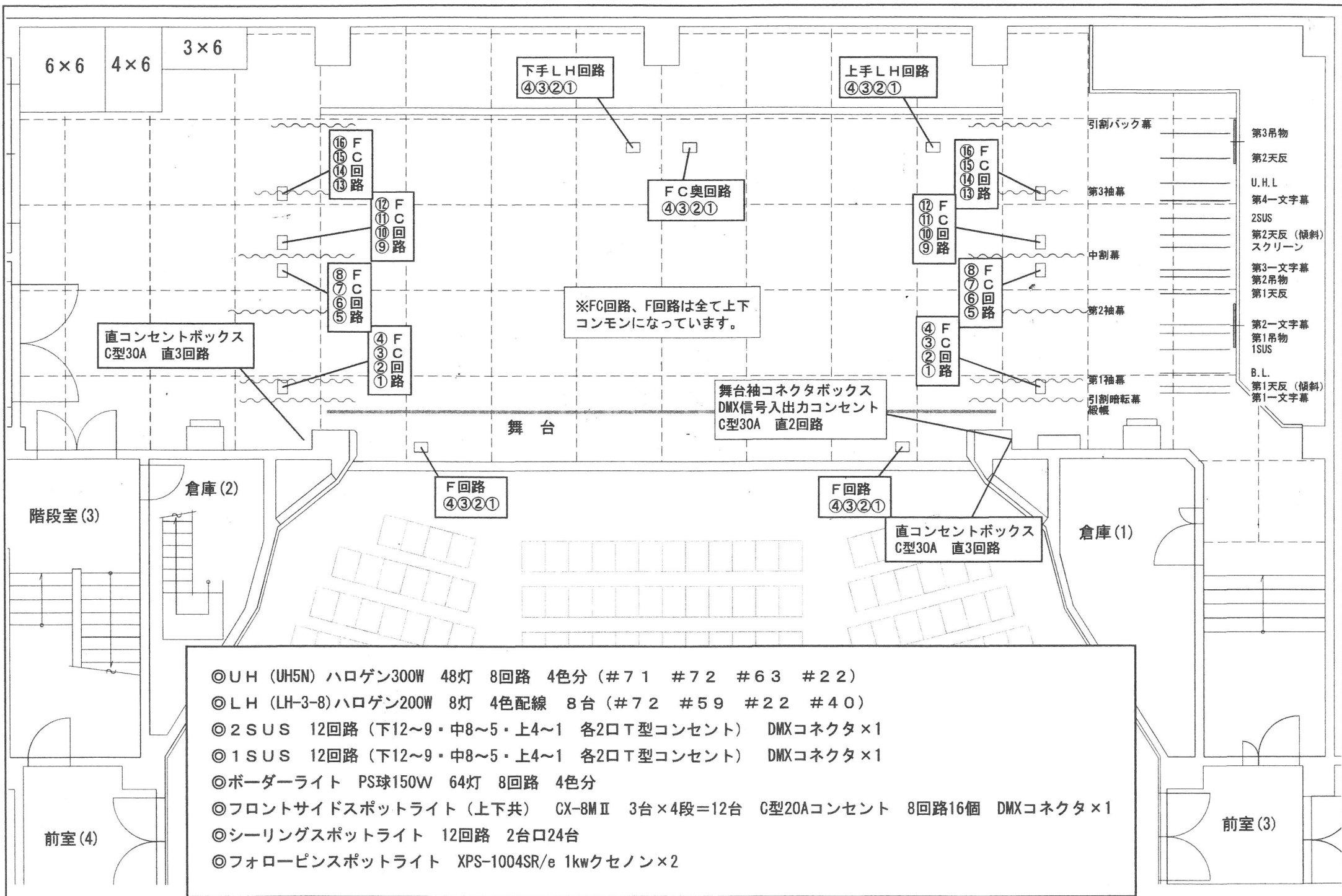
横浜市泉公会堂 照明回路図 (舞台ほか)
