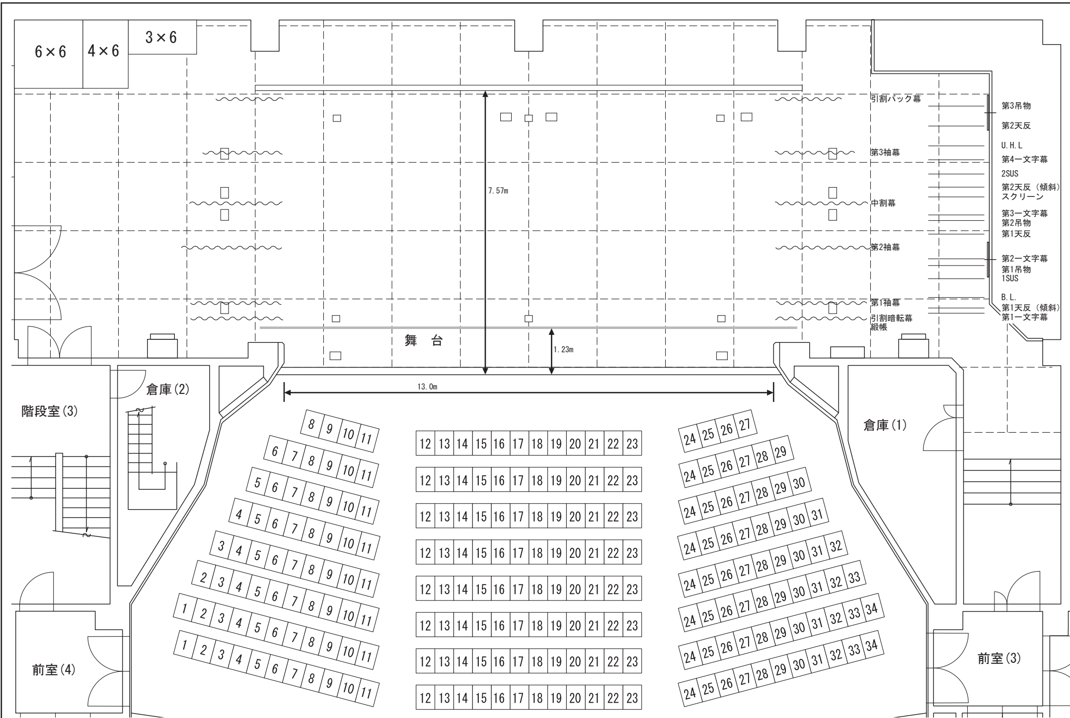
横浜市泉公会堂 講堂舞台平面図 1/100
