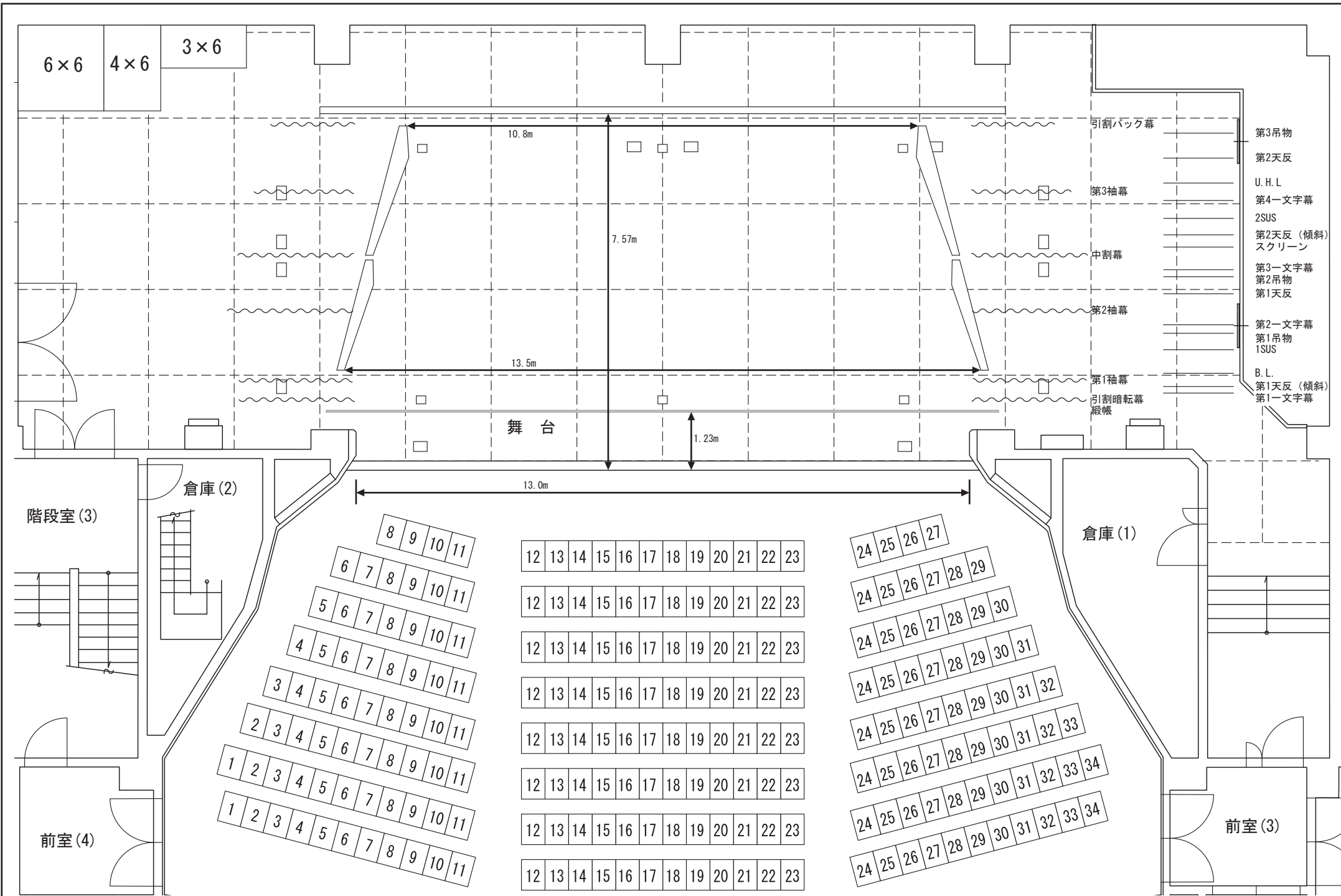
横浜市泉公会堂 講堂舞台平面図 (音響反射板仕様) 1/100
